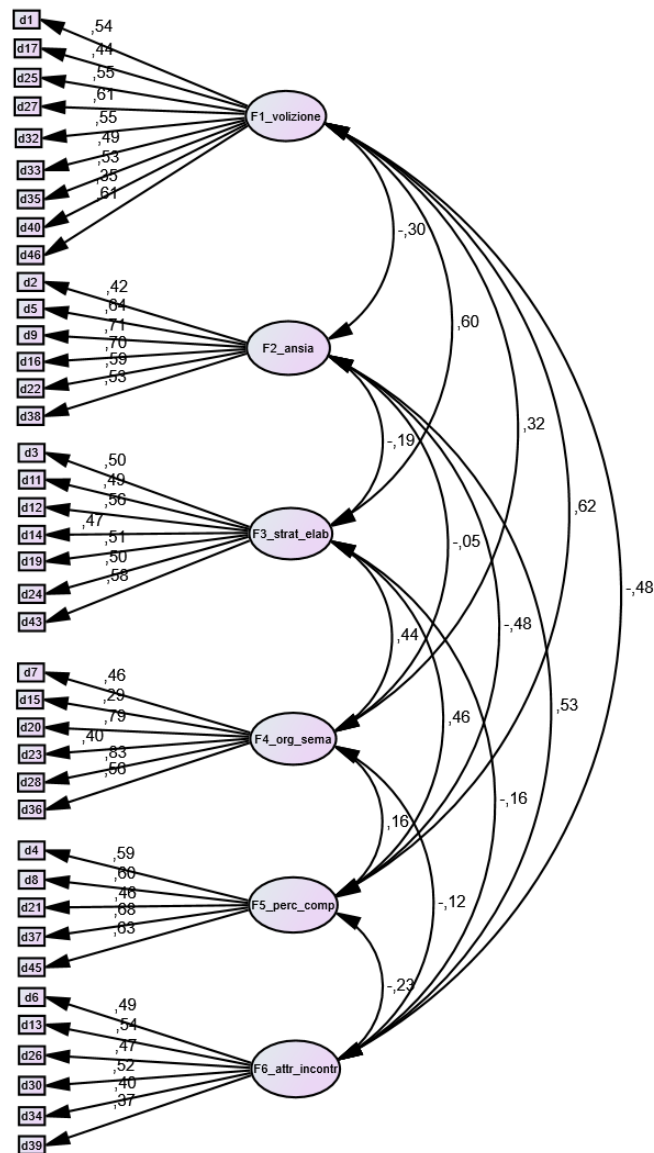
Figura 8: Saturazioni (valori standardizzati) e correlazioni dell'analisi fattoriale confermativa per la soluzione ottenuta con l'ACP.
